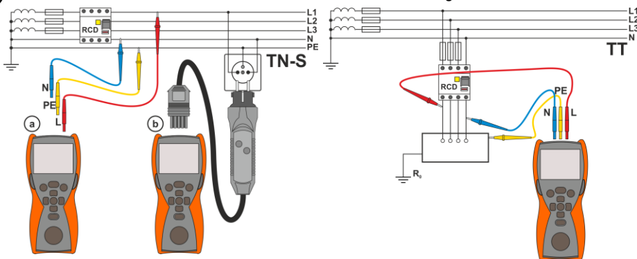
Medición en el circuito TN-S
